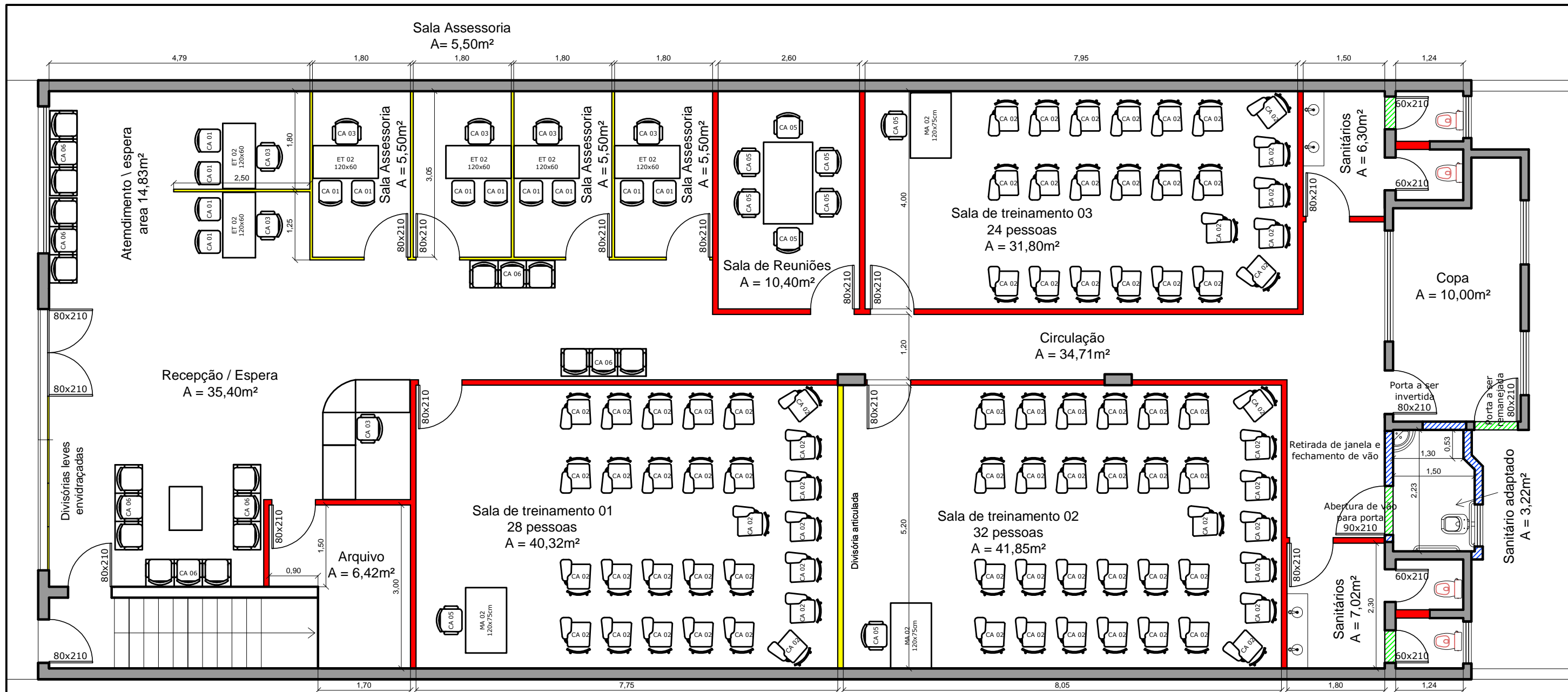
PLANTA BAIXA NOVA UNIDADE ZONA NORTE - Porto Alegre ESCALA: 1/75
